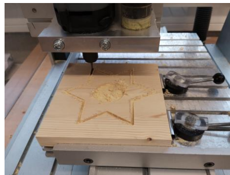
CNC-Fräse beim Ausfräsen des Sternes
